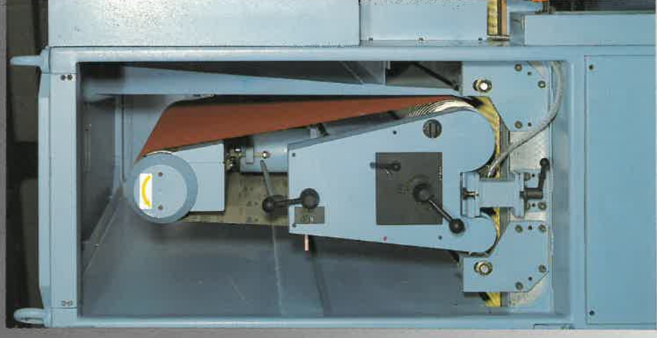
Kompaktes KOMBI-Schleifaggregat mit Kontaktwalze und Schleifschuh
