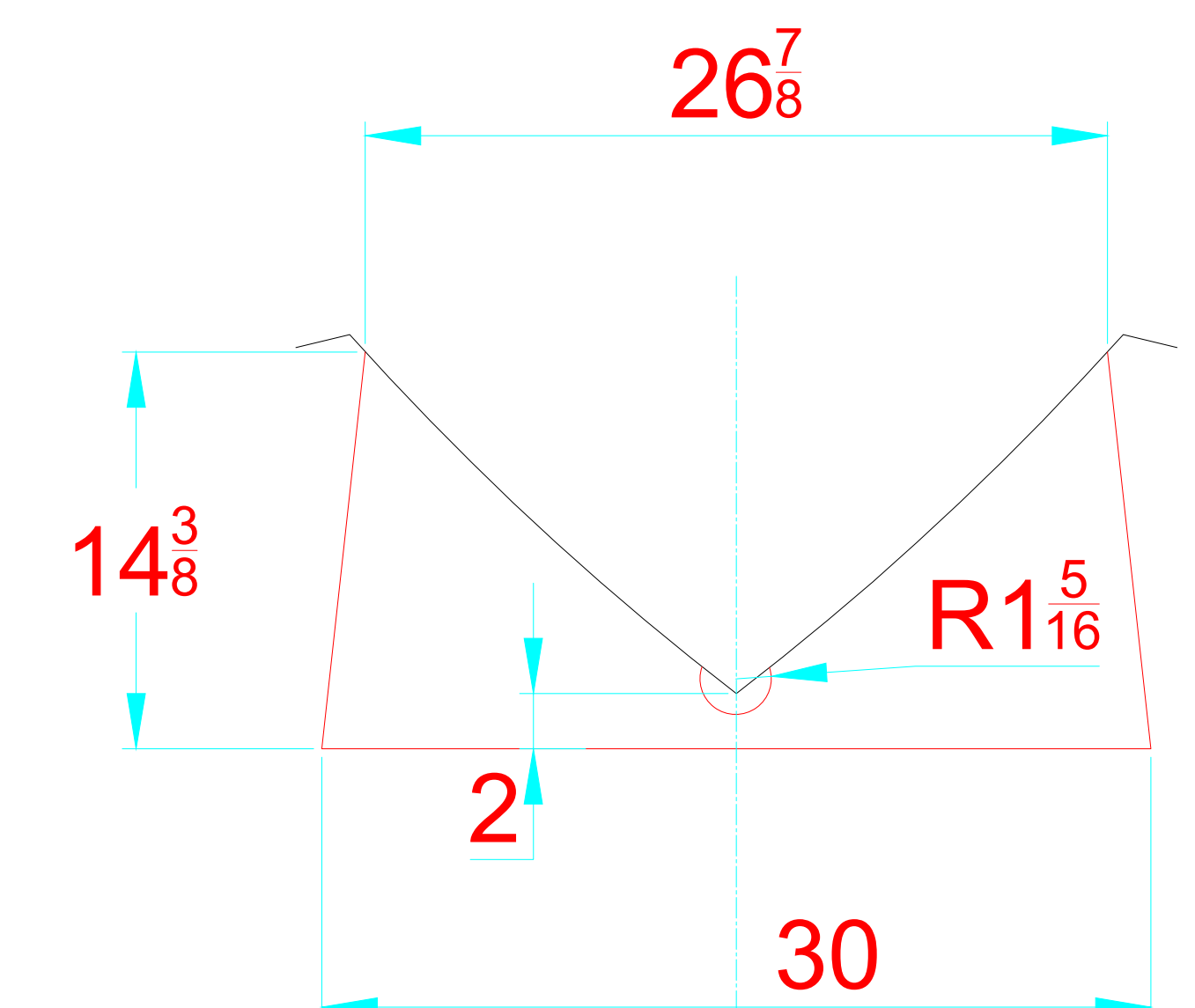
TRANSVERSAL SECTION "B" SECCION TRANSVERSAL "B"
