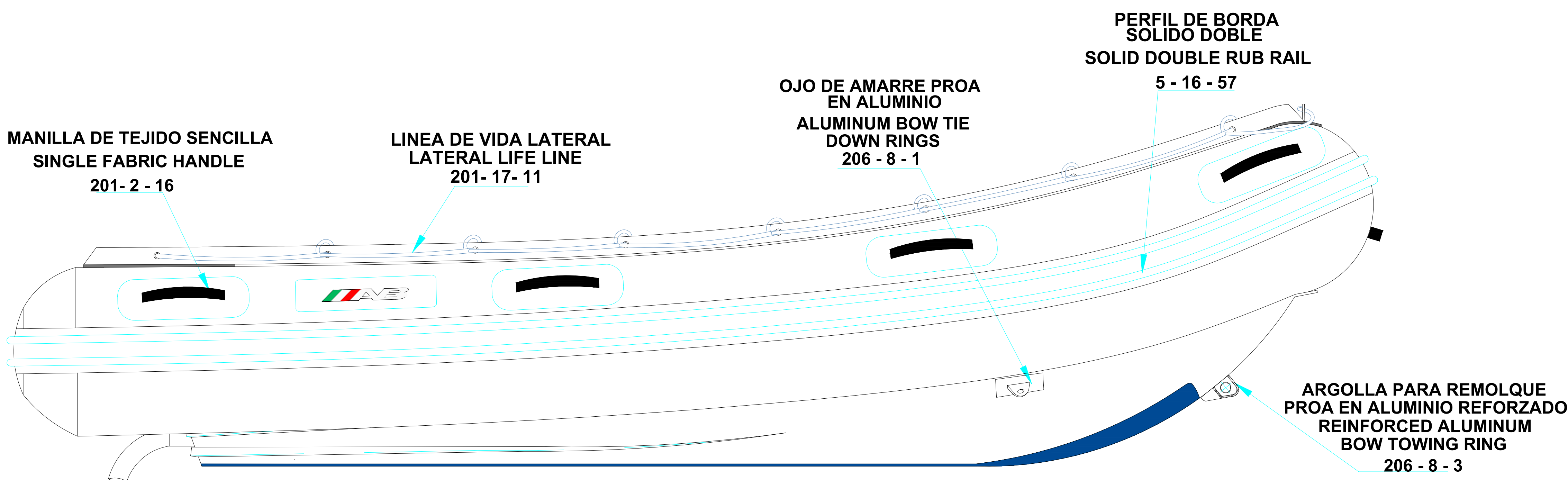
LONGITUDINAL PROFILE VISTA LATERAL
