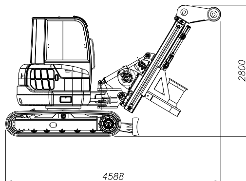
Dimensioni per il trasporto / Dimensions for transport Dimensions pour le transport / Dimensiones para el transporte
