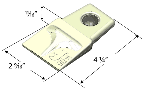
P/N 34070 (101)
