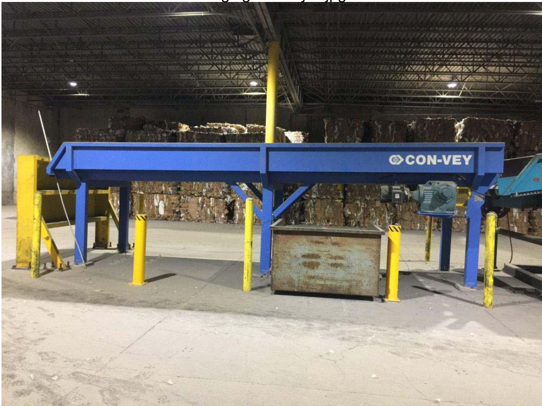
Staging Conveyor.jpg
