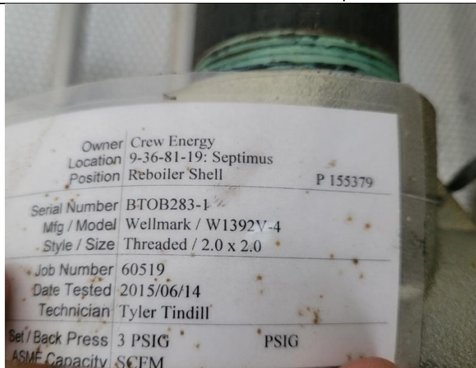
PSV tag
