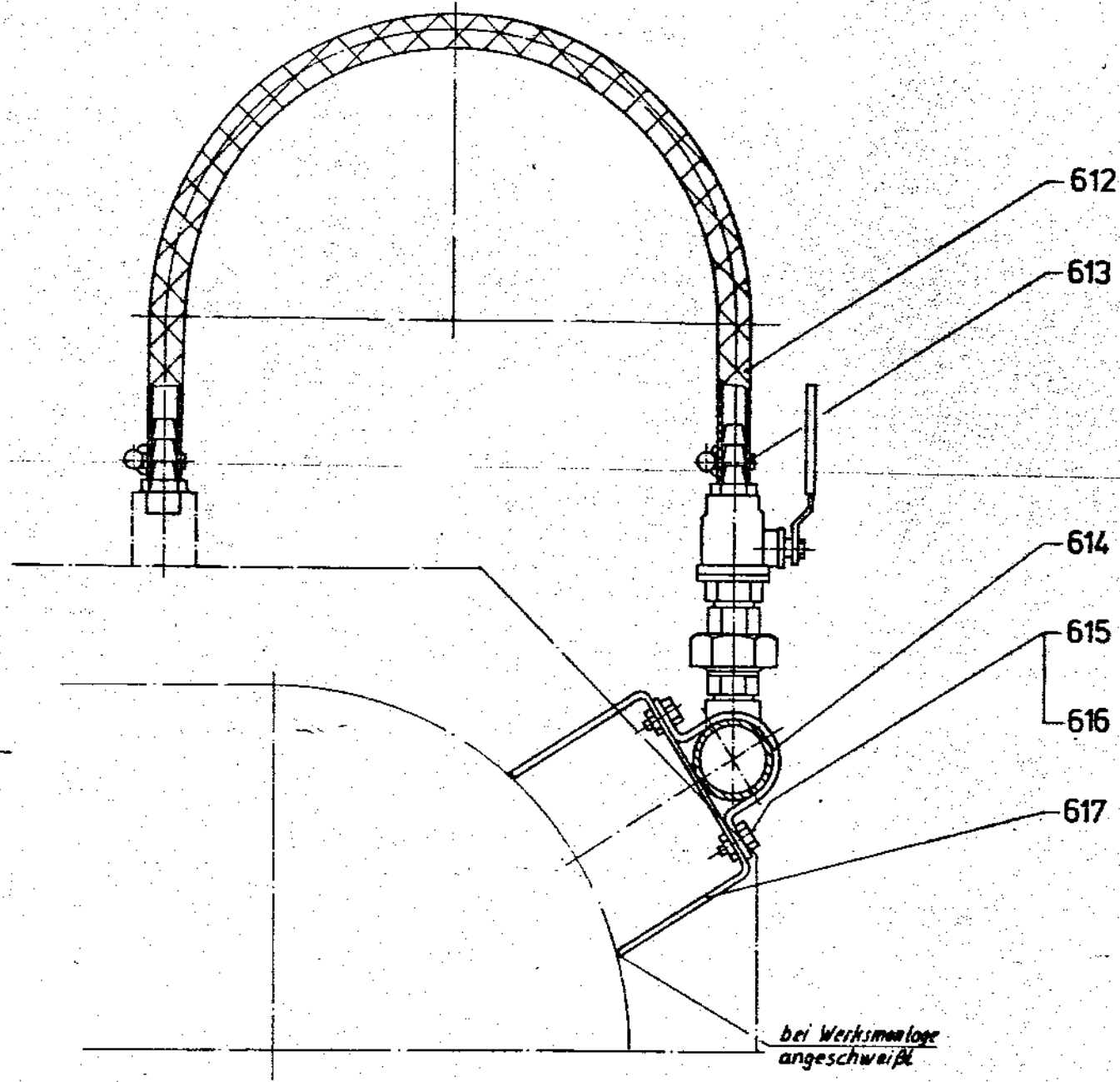
Schnitt A-A
