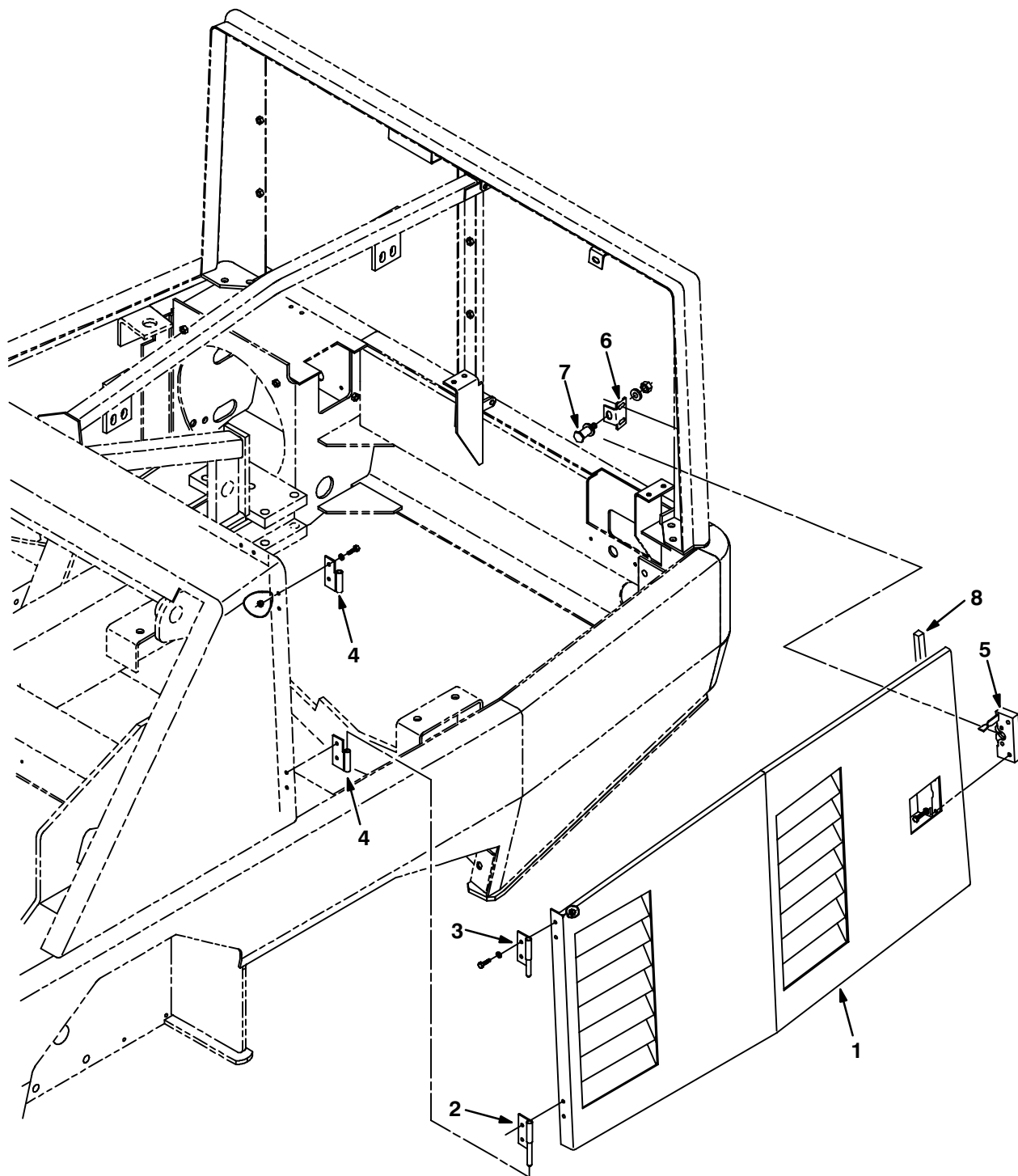
Fig. 11 – Engine Side Door Group
