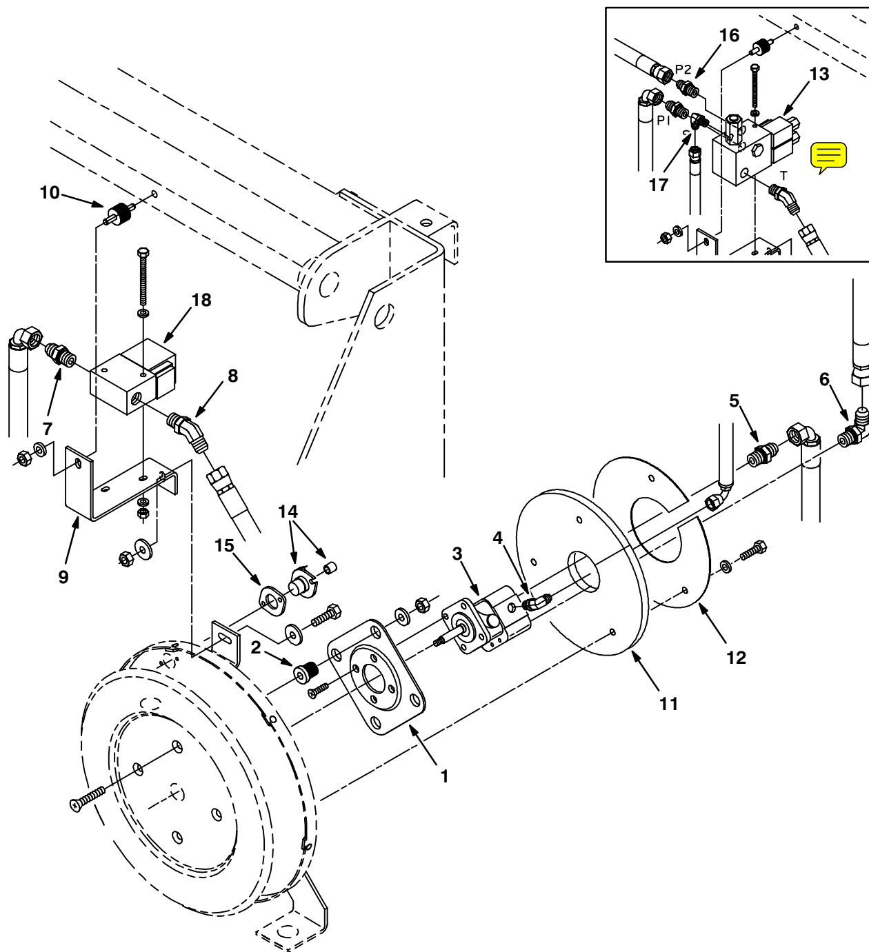
Fig. 66 – Vacuum Fan Motor Group
