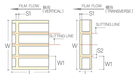
四线密封 4 Lane Seal
