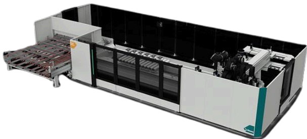
Biesse Rover Multi Pro W G
