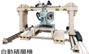
自動積層機 Auto lay-up machine 自动积层机
