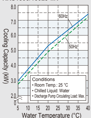
RKS1503/1502J-MV
