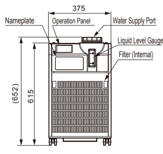
RKS402J-MVW
