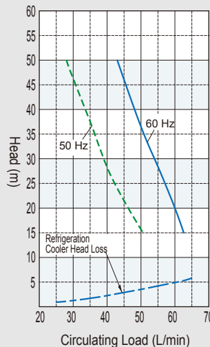
RKE2200B1-V/VW
