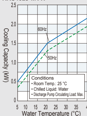
RKS402J-MVW
