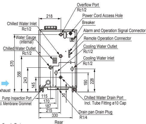
RKS402J-MVW
