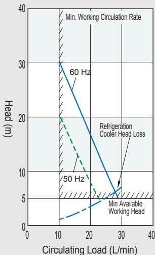
RKE750A1-V
