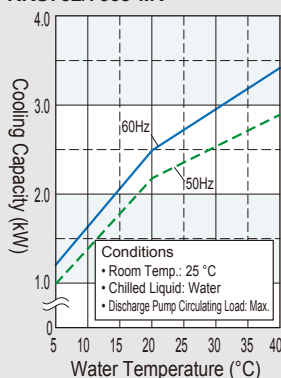
RKS752/753J-MV
