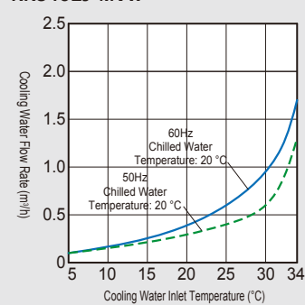
RKS402J-MVW
