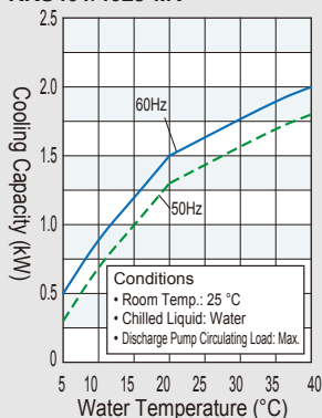
RKS401/402J-MV
