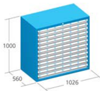
MODELO GR/TX-1000
