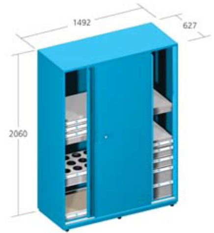
MODELO APC/TX-2000
