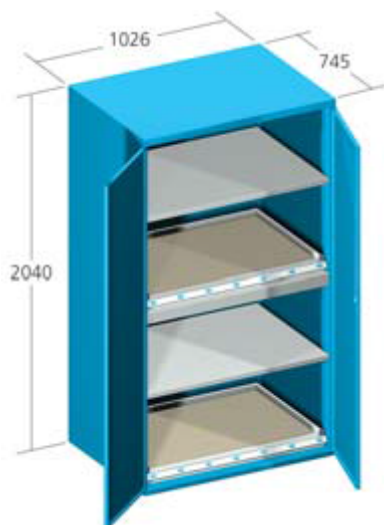
MODELO P/GR-2000
