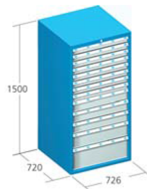
MODELO SP-1500
