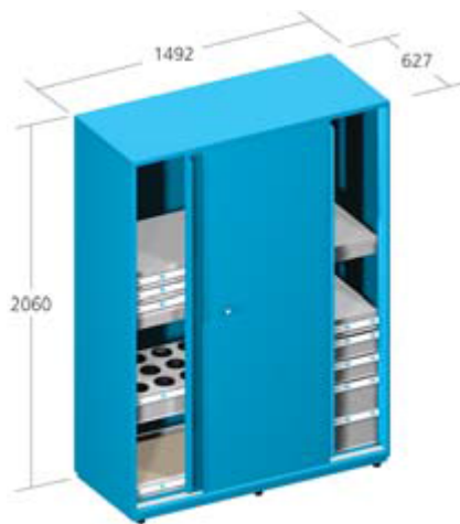
MODELO APC/TX-1250
