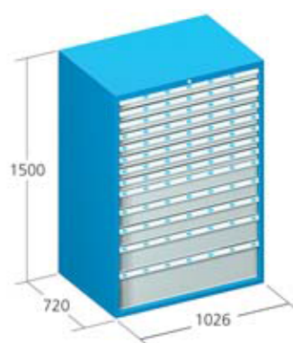
MODELO GR-1500
