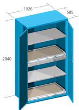
MODELO P/GR/TX-2000
