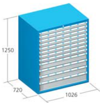
MODELO GR-1250
