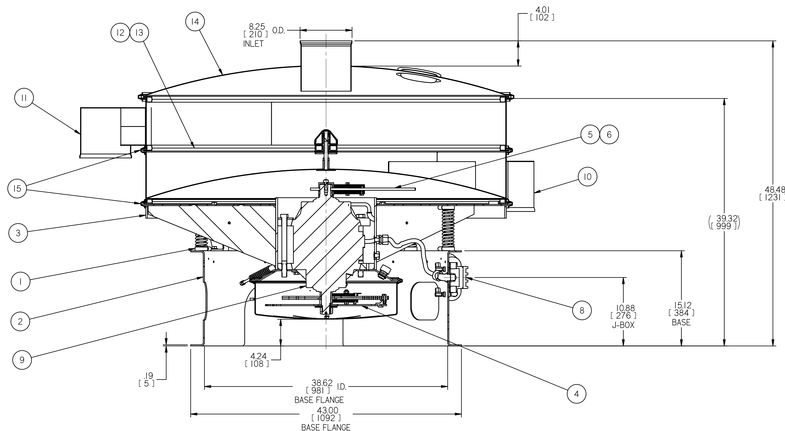
SECTION A-A 1:8
