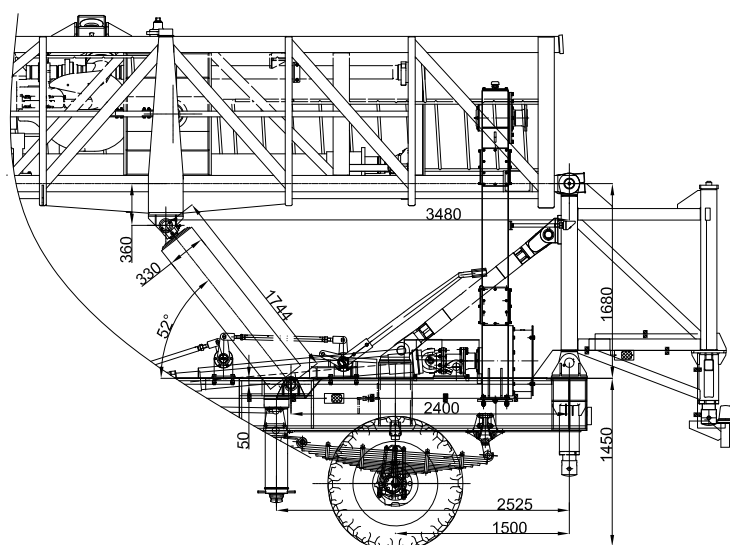
Geometria de rabatere 1:25
