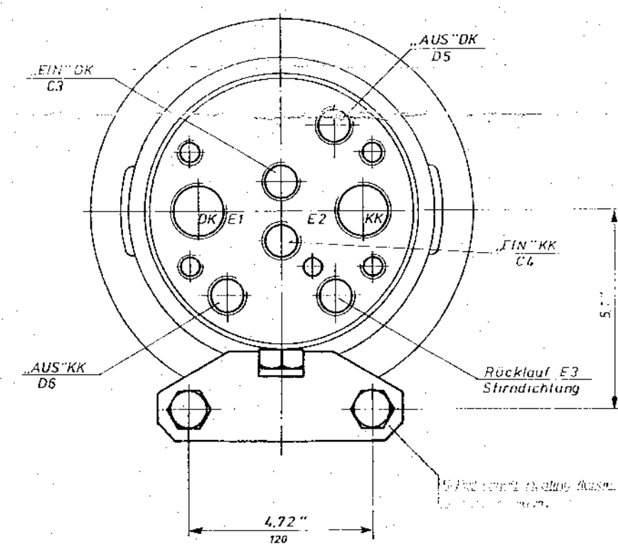
Section G-H Schnitt
