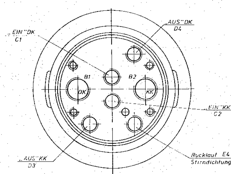
Section E-F Schnitt
