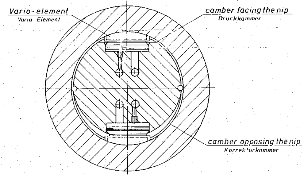
Section I-K Schnitt
