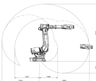
IRB 6700-175/3.05
