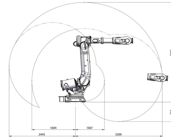
IRB 6700-150/3.20
