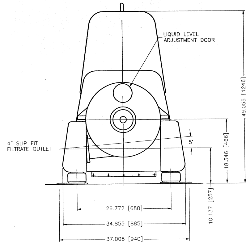
VIEW A-A
