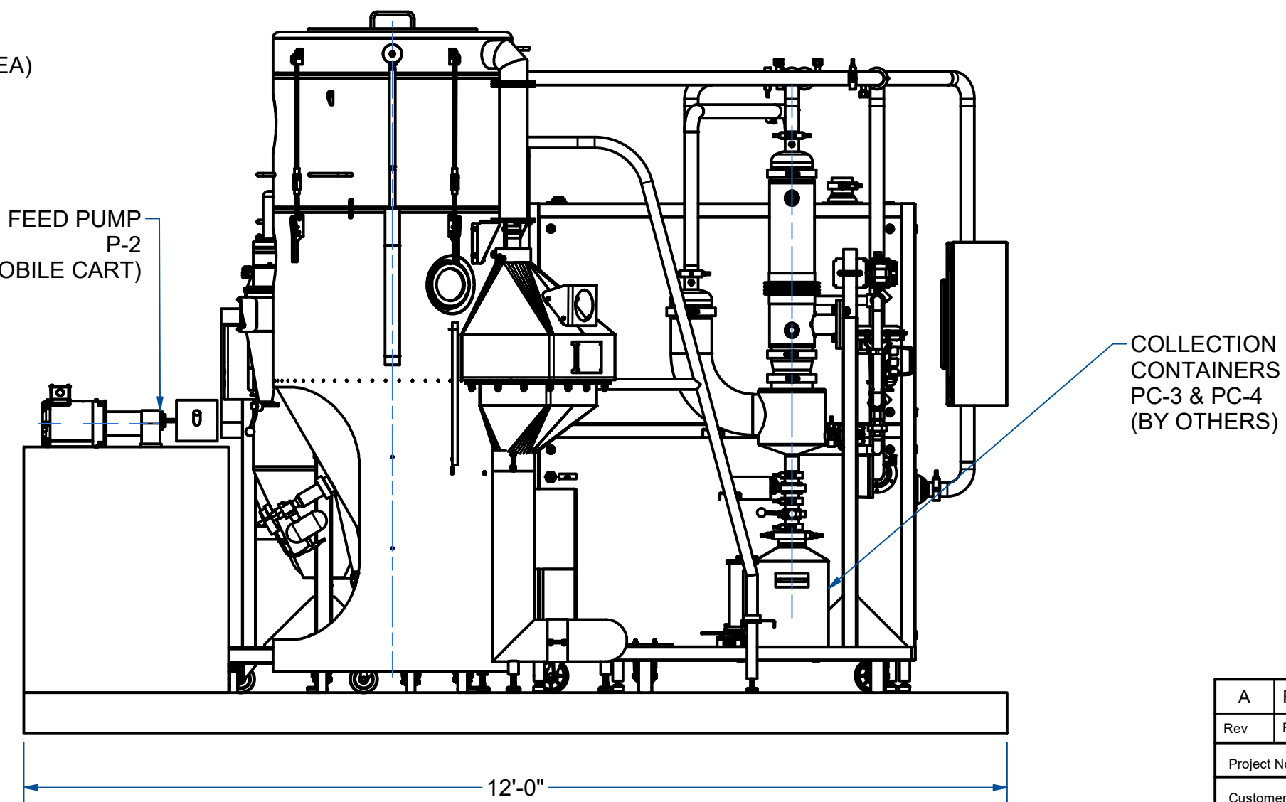
SIDE VIEW SCALE: 1 / 20
