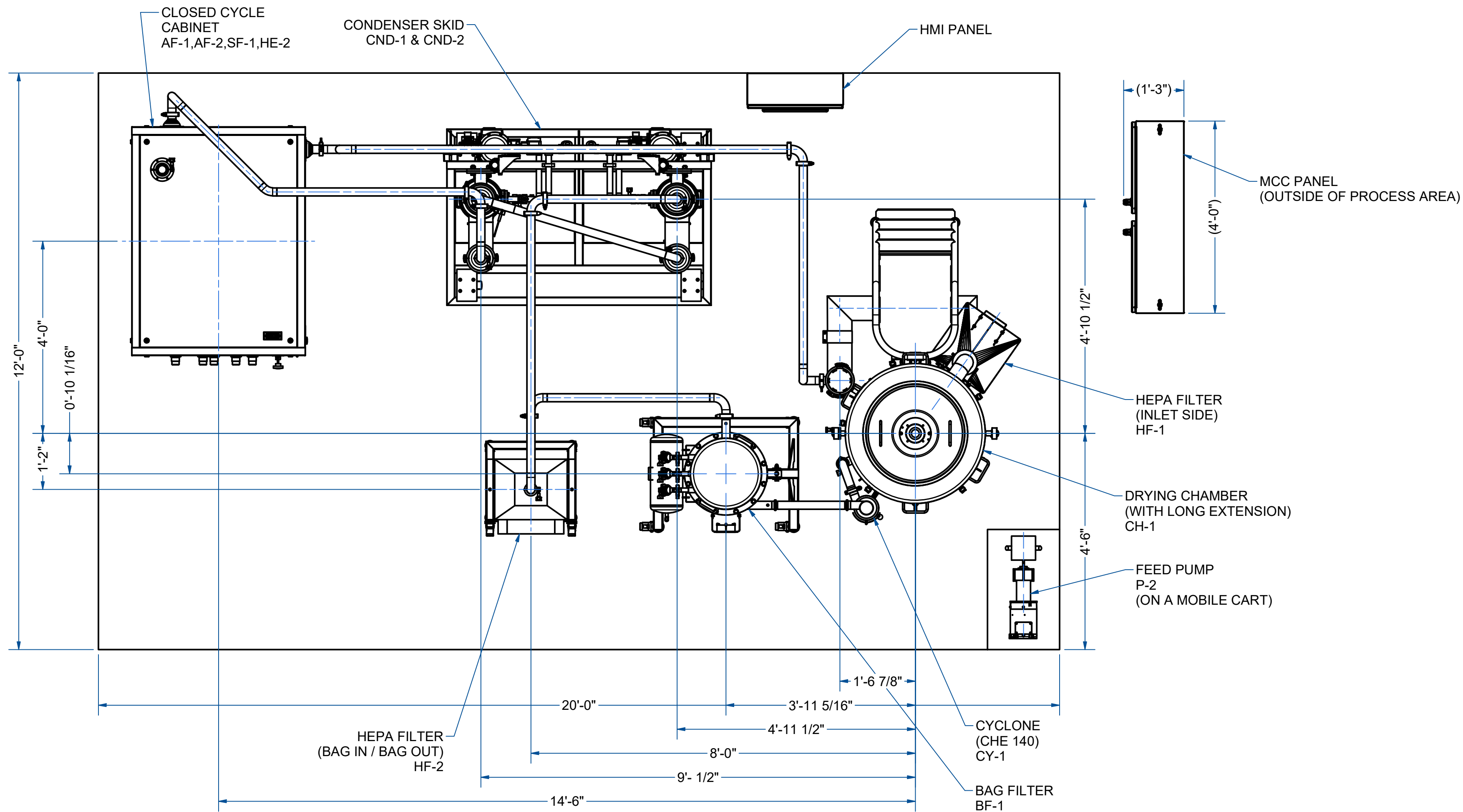
TOP VIEW SCALE: 1 / 20
