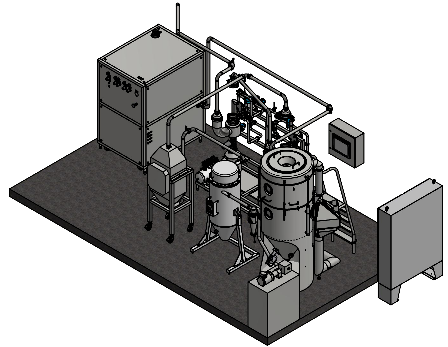
ISOMETRIC VIEW SCALE: 1 / 32
