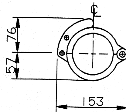
COUPLING DIMENSIONS
