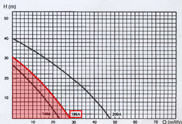
Fig. 2. Kapacitetsdiagram.
