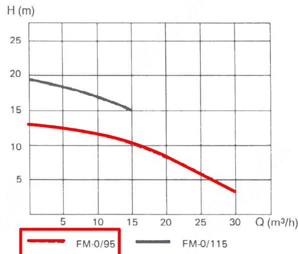
Fig. 2. Kapacitetsdiagram.
