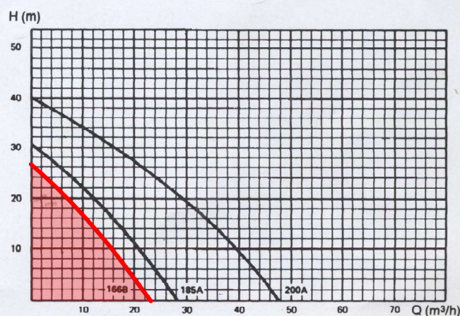
Fig. 2. Kapacitetsdiagram.
