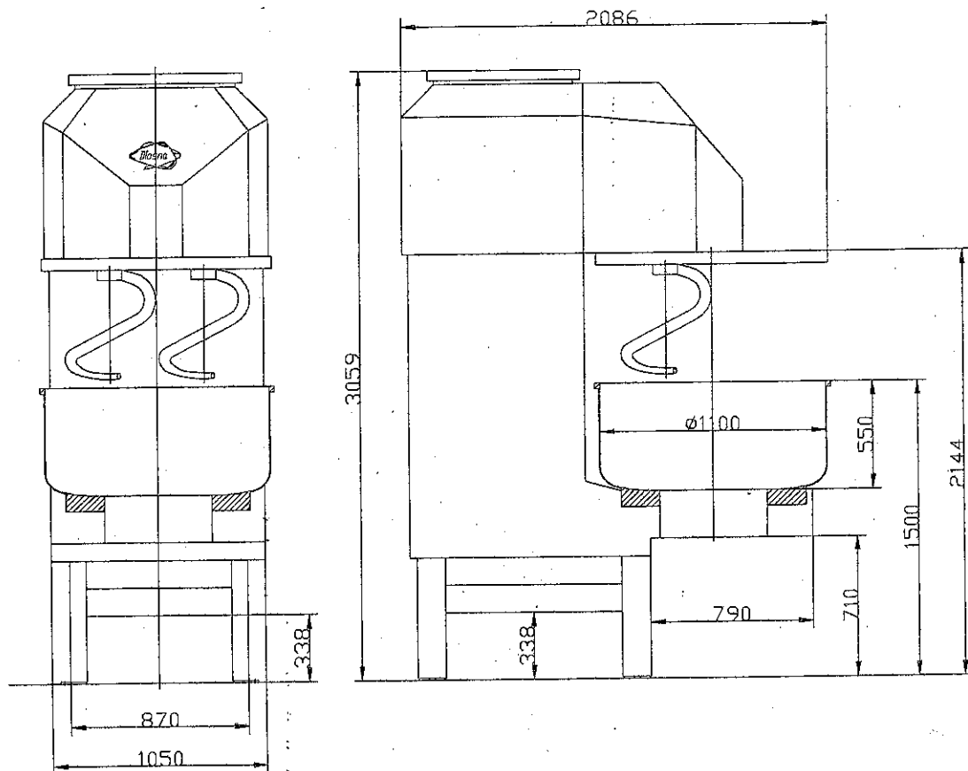
Bild 2-3: Abmessungen
