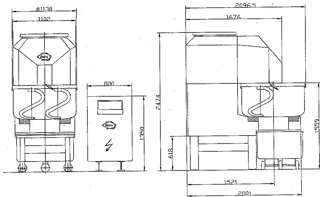
Bild 2-2: Abmessungen
