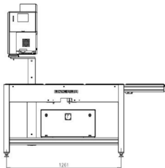
GLM-Emaxx_50_frontal
