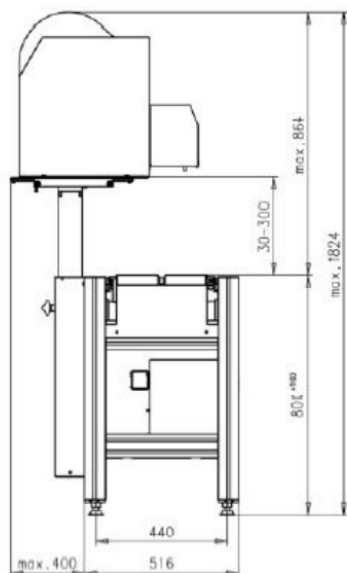
GLM-Emaxx_50_seitlich
