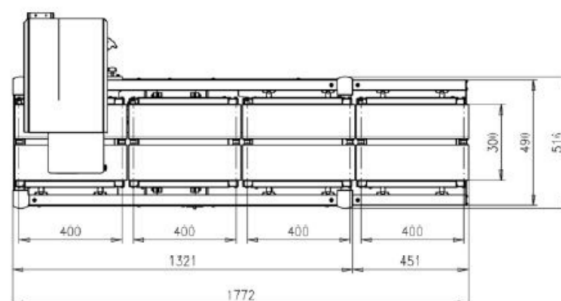
GLM-Emaxx_50_draufsicht
