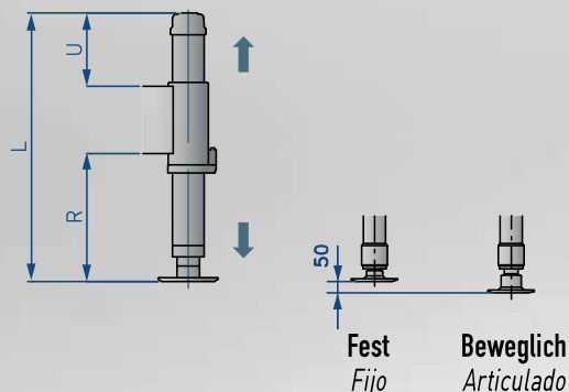
K-System für Höhenverstellung K-Sistema de regulación en altura
